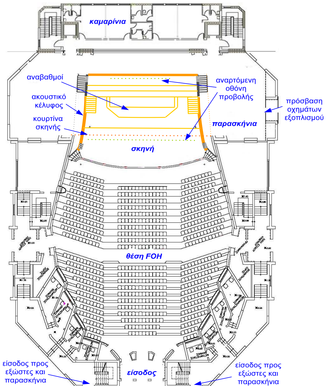
Σχήμα 1: κάτοψη του επιπέδου της πλατείας του μεγάλου Αμφιθεάτρου του Συνεδριακού – Πολιτιστικού Κέντρου
